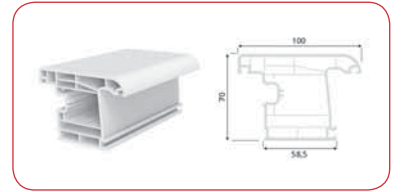
DIŞA AÇILIR KİLİTLİ KAPI PROFİLİ
