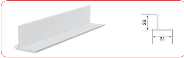
DAR AŞİMETRİK T PROFİLİ
