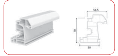
DAMLALIKLI KANAT PROFİLİ
