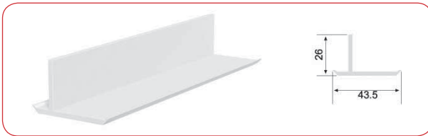
GENİŞ AŞİMETRİK T PROFİLİ
