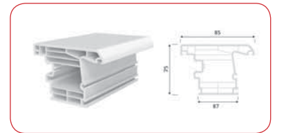
75 DIŞA AÇILIR KİLİTLİ KAPI PROFİLİ
