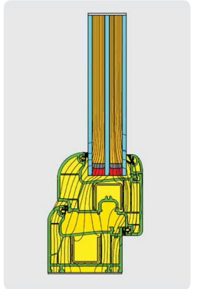
PENCERE ISI AKIŞ DIYAGRAMI UF:1,02 W/M 2 *K UW: 1,05 W/M 2 *K
